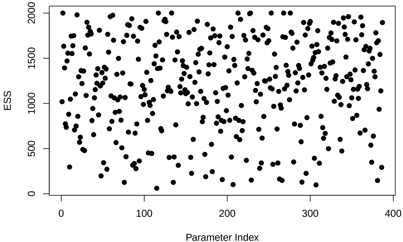
ESS vs Parameter Index
