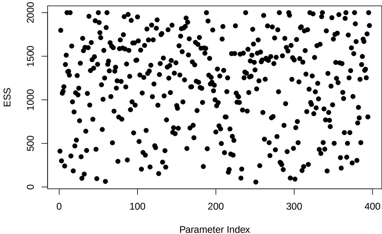
ESS vs Parameter Index
