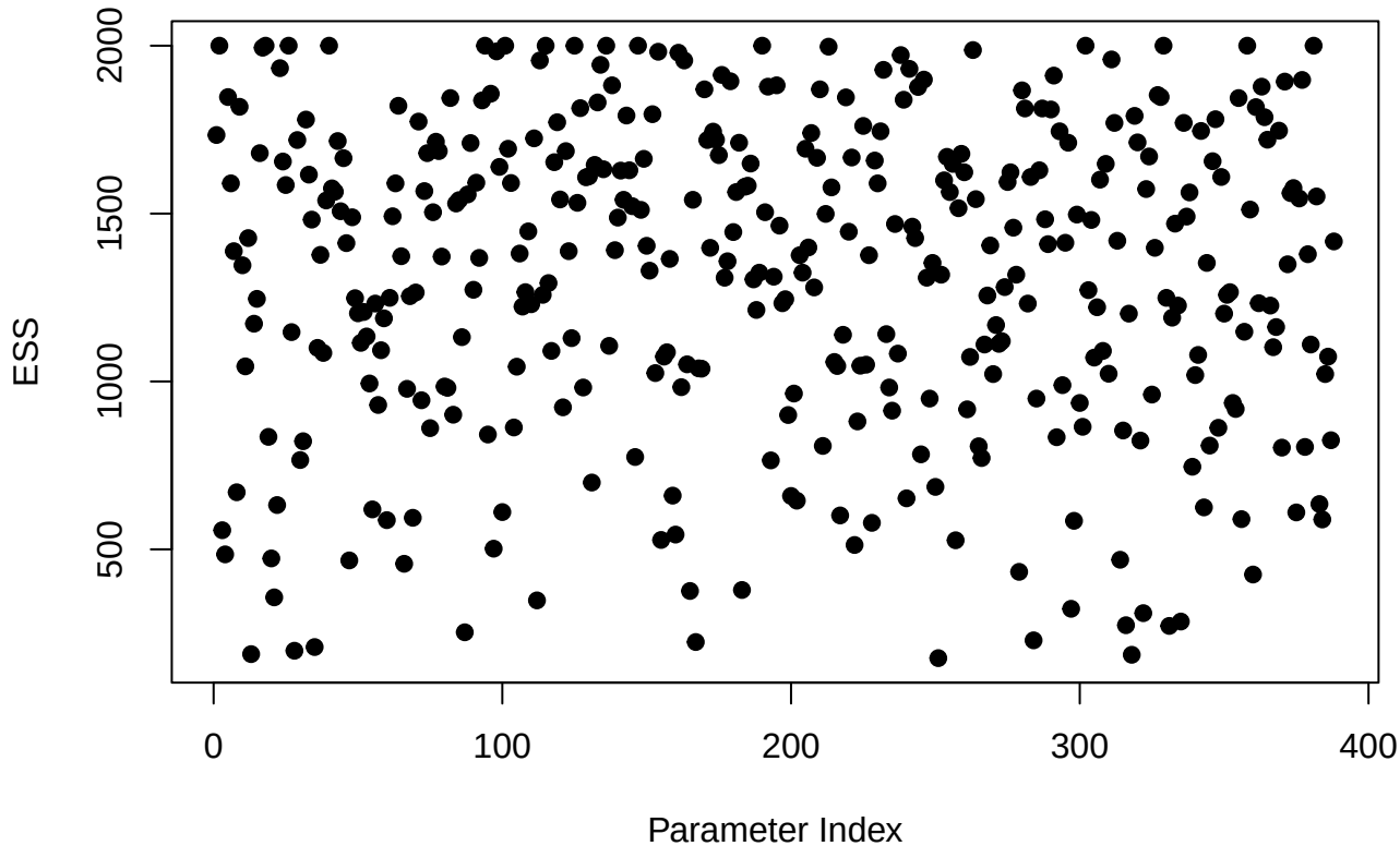
ESS vs Parameter Index
